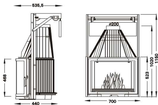
Krbová vložka Uniflam 700 Prizmat horní otevírání
