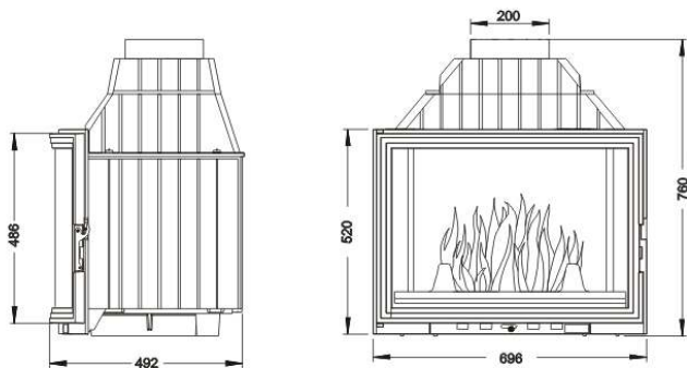
Krbová vložka Uniflam 700 Panorama
